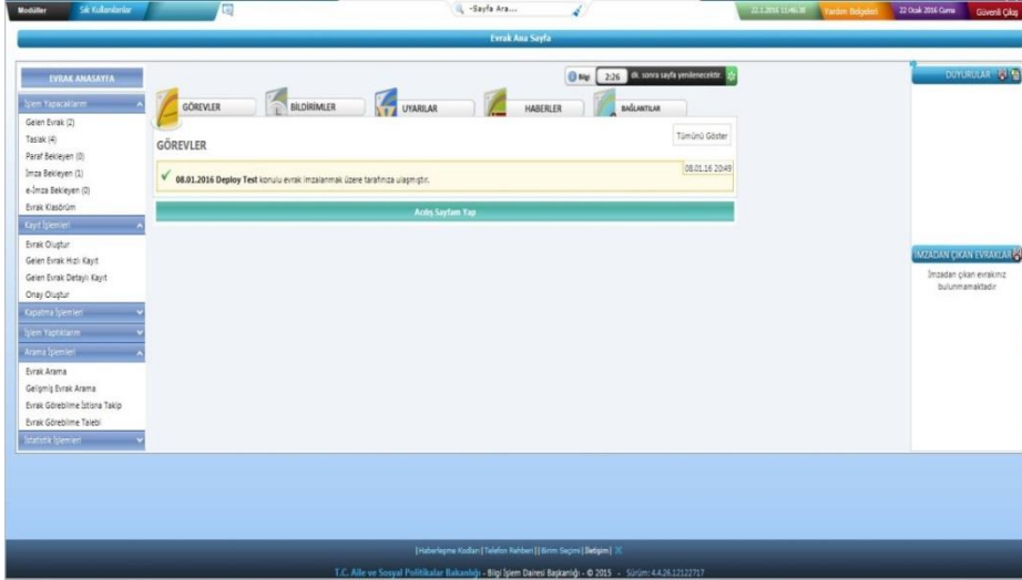
Şekil 3: EBYS ekranı
